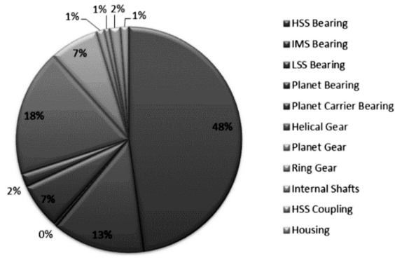
Fig. 2. Wind turbine gearbox failures, divided according to the component [L. 2] Rys. 2. Udział uszkodzeń poszczególnych elementów przekładni w ogólnej liczbie awarii [L. 2]
