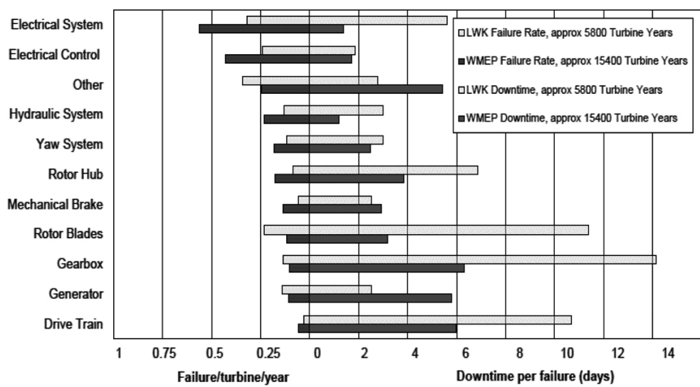
Fig. 1. Failure rate and downtime of specific systems [L. 1] Rys. 1. Częstotliwość uszkodzeń oraz przestoje spowodowane przez awarie poszczególnych podzespołów [L. 1]
