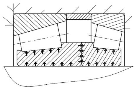
Fig. 3. The mechanism of preload generation, based on interference between the bearing and the shaft [L. 3] Rys. 3. Sposób wywierania napięcia wstępnego poprzez wcisk pomiędzy wałem a pierścieniem łożyska [L. 3]
