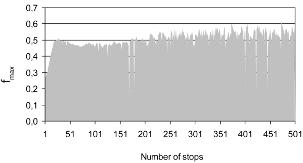
Fig. 6. The change of the maximum friction coefficient (f max ) obtained using the T-33 inertia dynamometer Rys. 6. Przebieg maksymalnego współczynnika tarcia (f max ) uzyskany na stanowisku T-33
